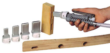
Obj.č.: 228-232 Popis: tryska na dlabané spoje
